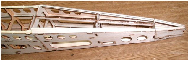
22. Glue rear bottom cover(F53).
